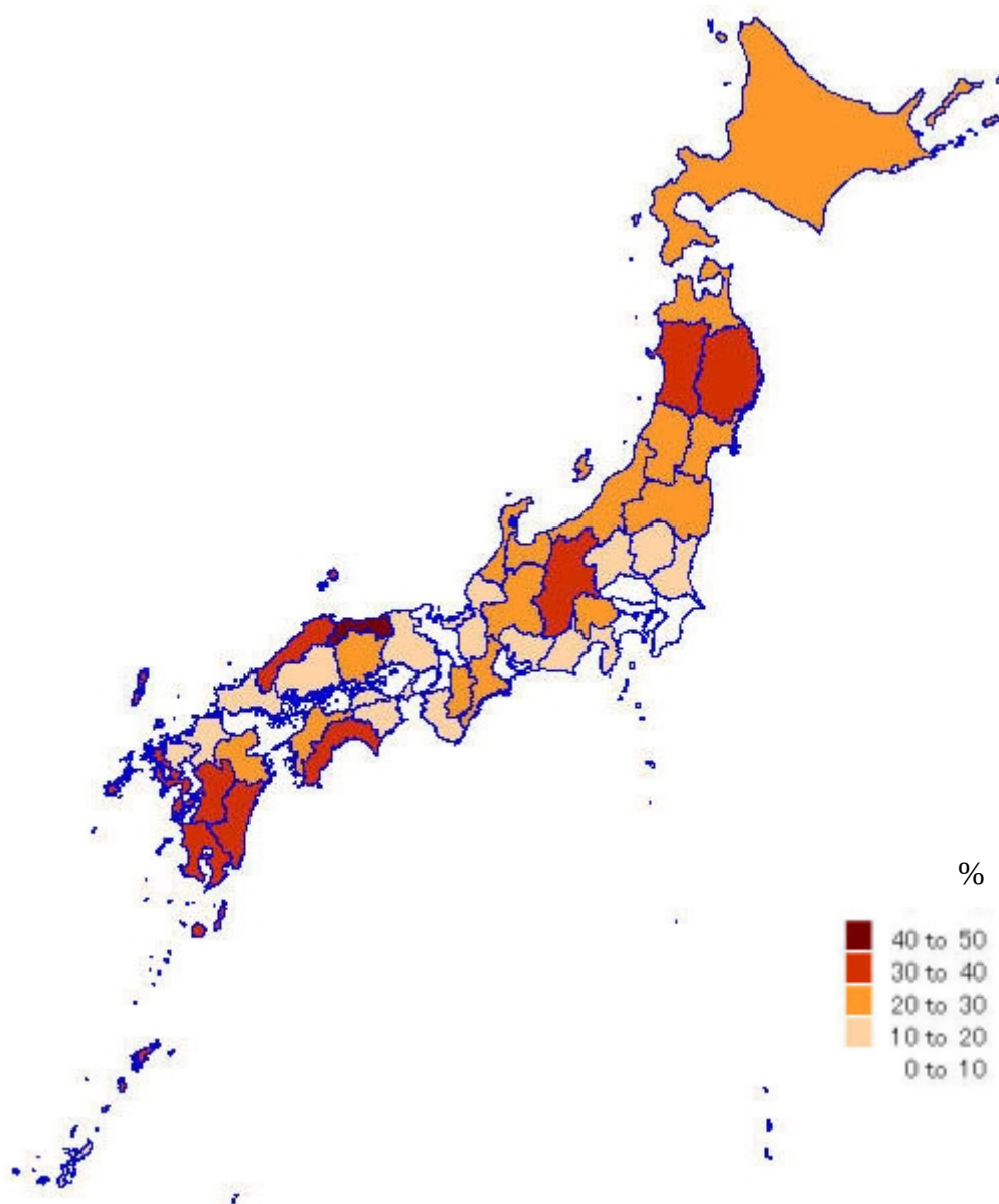
図2-2-3: 各都道府県における、1997年11月時点の郵便局に占める簡易郵便局の比率。
