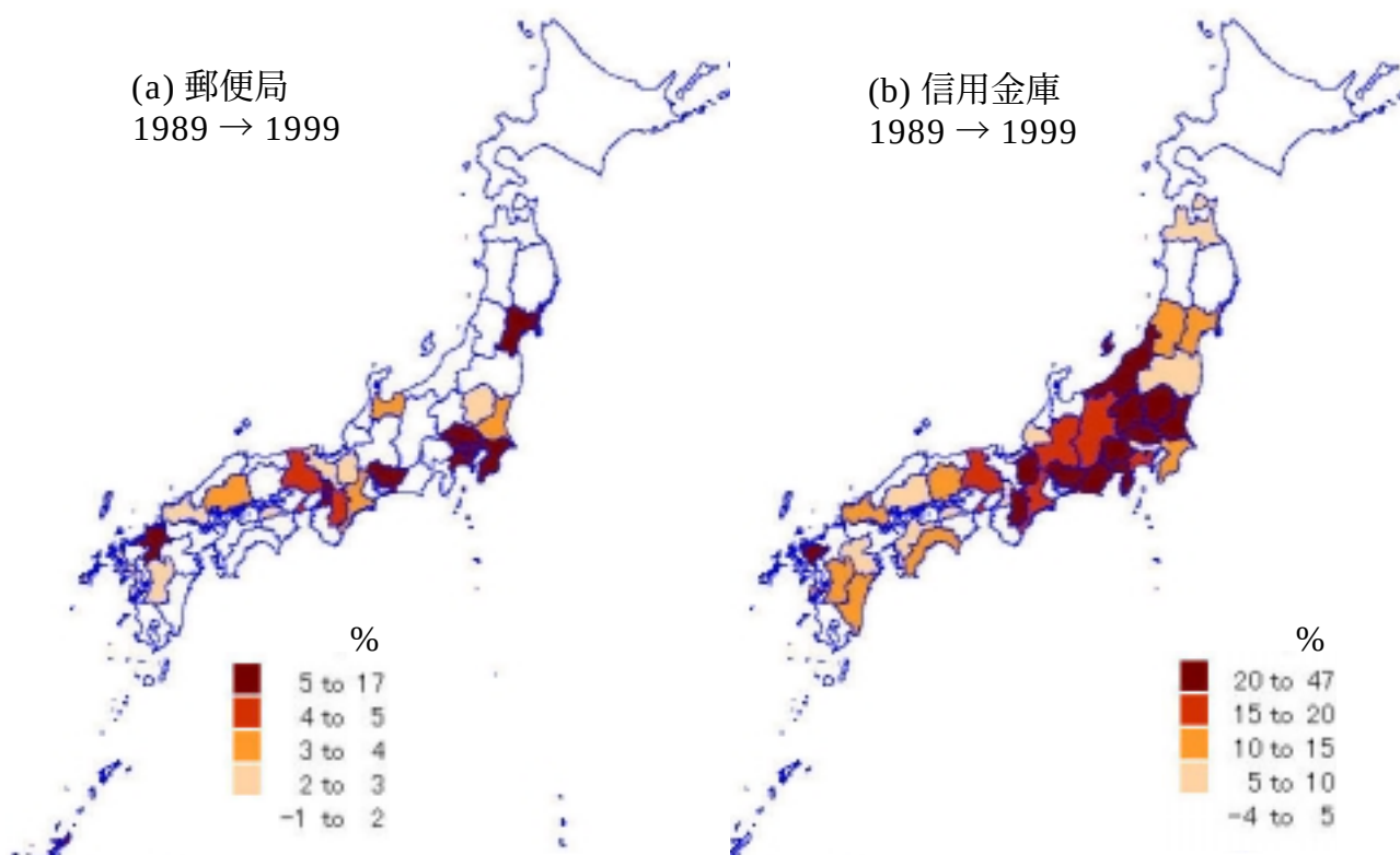
図2-2-2: 各都道府県における、1989年3月から1999年3月にかけての拠点数の伸び率: (a) 郵便局、(b)信用金庫。
